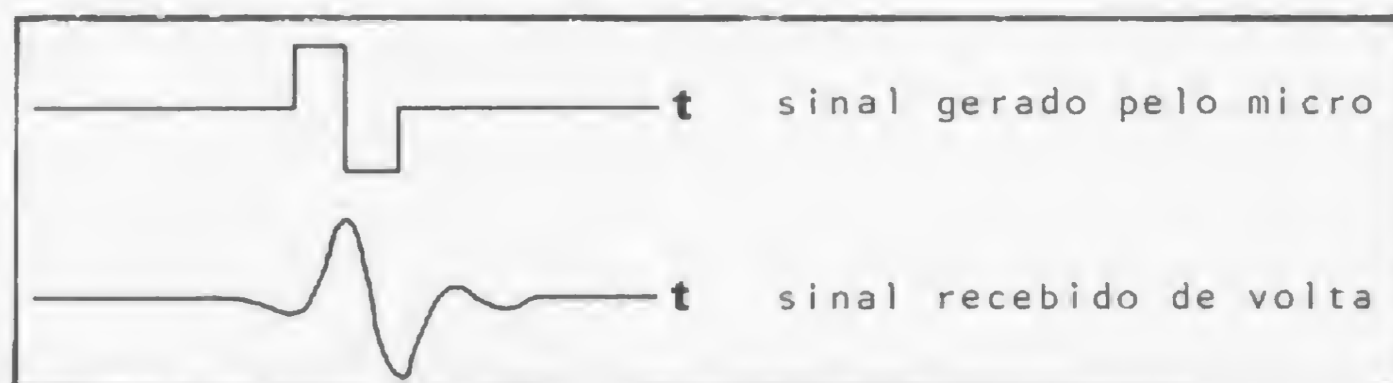
Figura 2 — Distorção no sinal.
